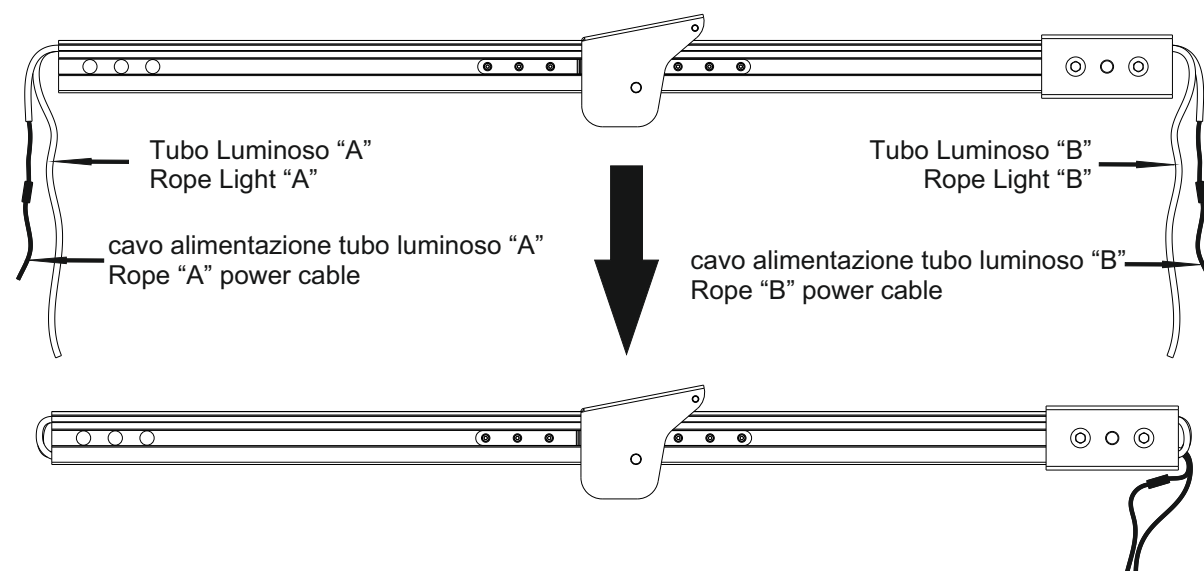
Installazione del kit luci su asta di dimensioni 100x66, in presenza dell'AJ01130
