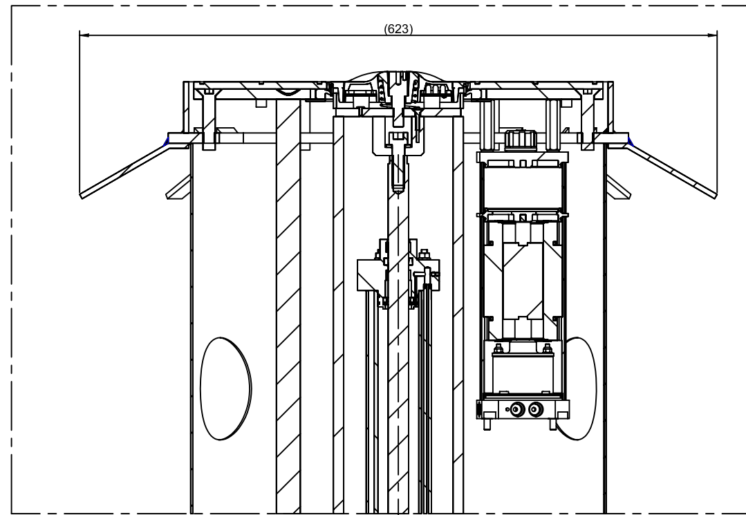
DETTAGLIO C
