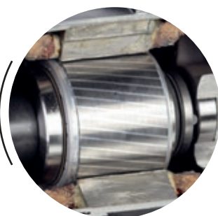
EMBAYAGE À DOUBLE DISQUE À BAIN D'HUILE (PASS2500)
