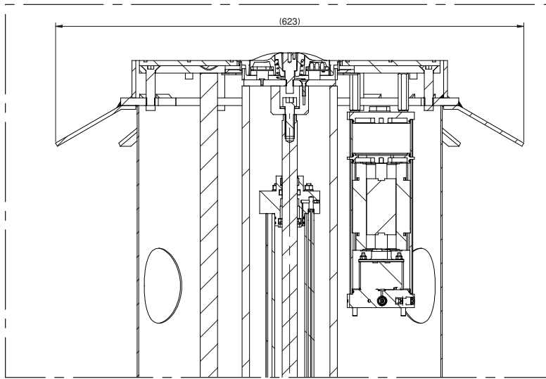
DETTAGLIO C
