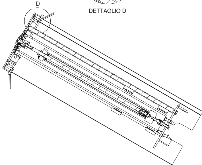
SEZIONE B-B
