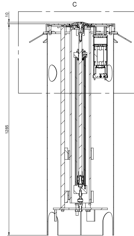
SEZIONE A-A
